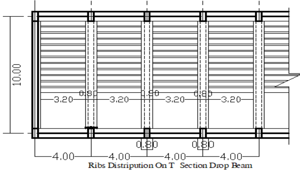
شكل 3. طريقة توزيع الأحمال على الجسور حيث توزيع الحمل عرضيا على الجسور الطويلة بالاتجاه (A)
