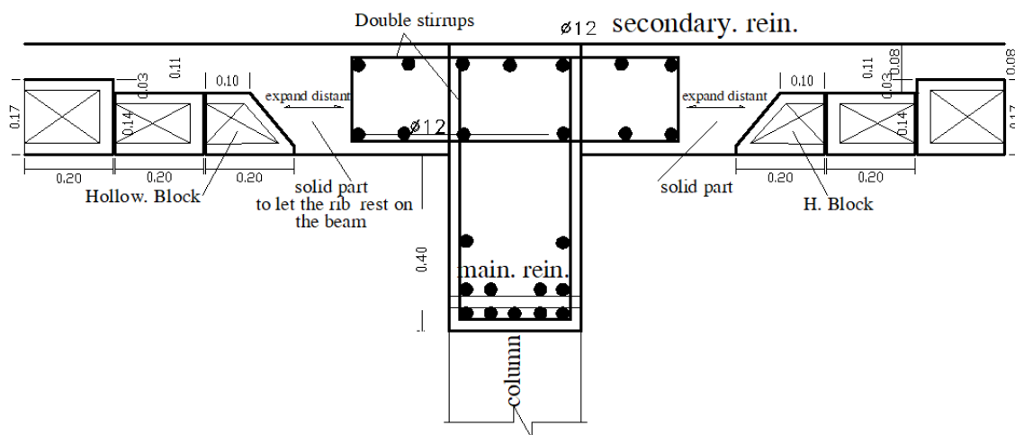
شكل 8. بين تفاصيل تنفيذ جسر قطاع (T) مع اختلاف ارتفاع طوب العقدة
