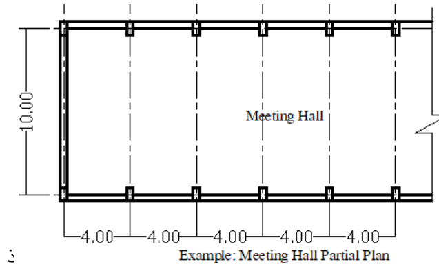
شكل 2. مثال على صالة مستطيلة التصميم بدون أعمدة وسطية
