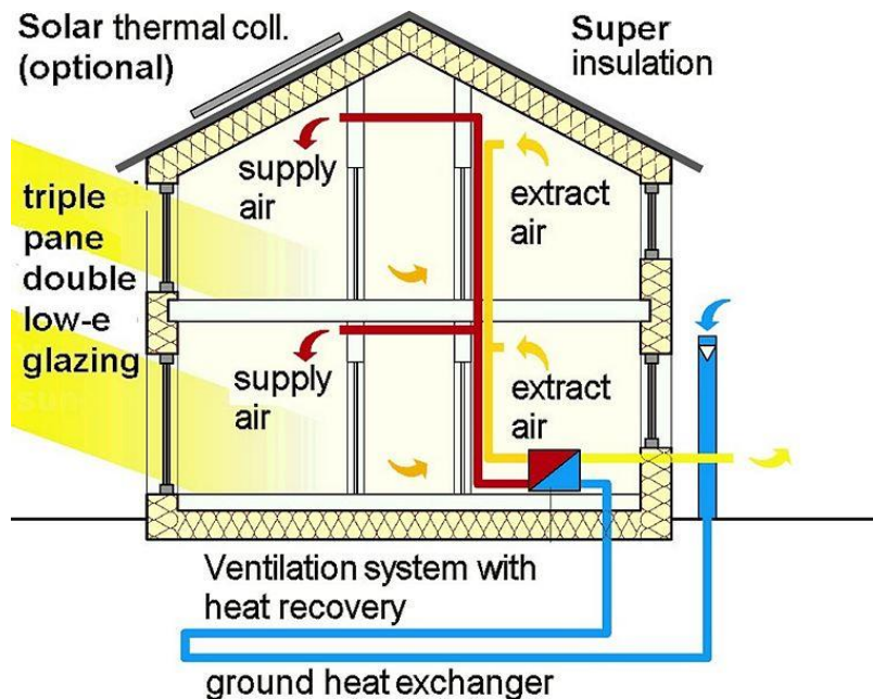
مقطع عرضي لمنزل سلبي يستخدم تقنيات مختلفة من أجل توفير الطاقة
