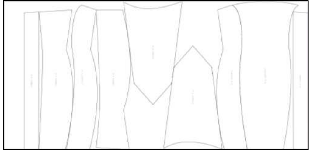
شكل (7) رسم باترون التصميم العاشر (اعداد الباحثين)
